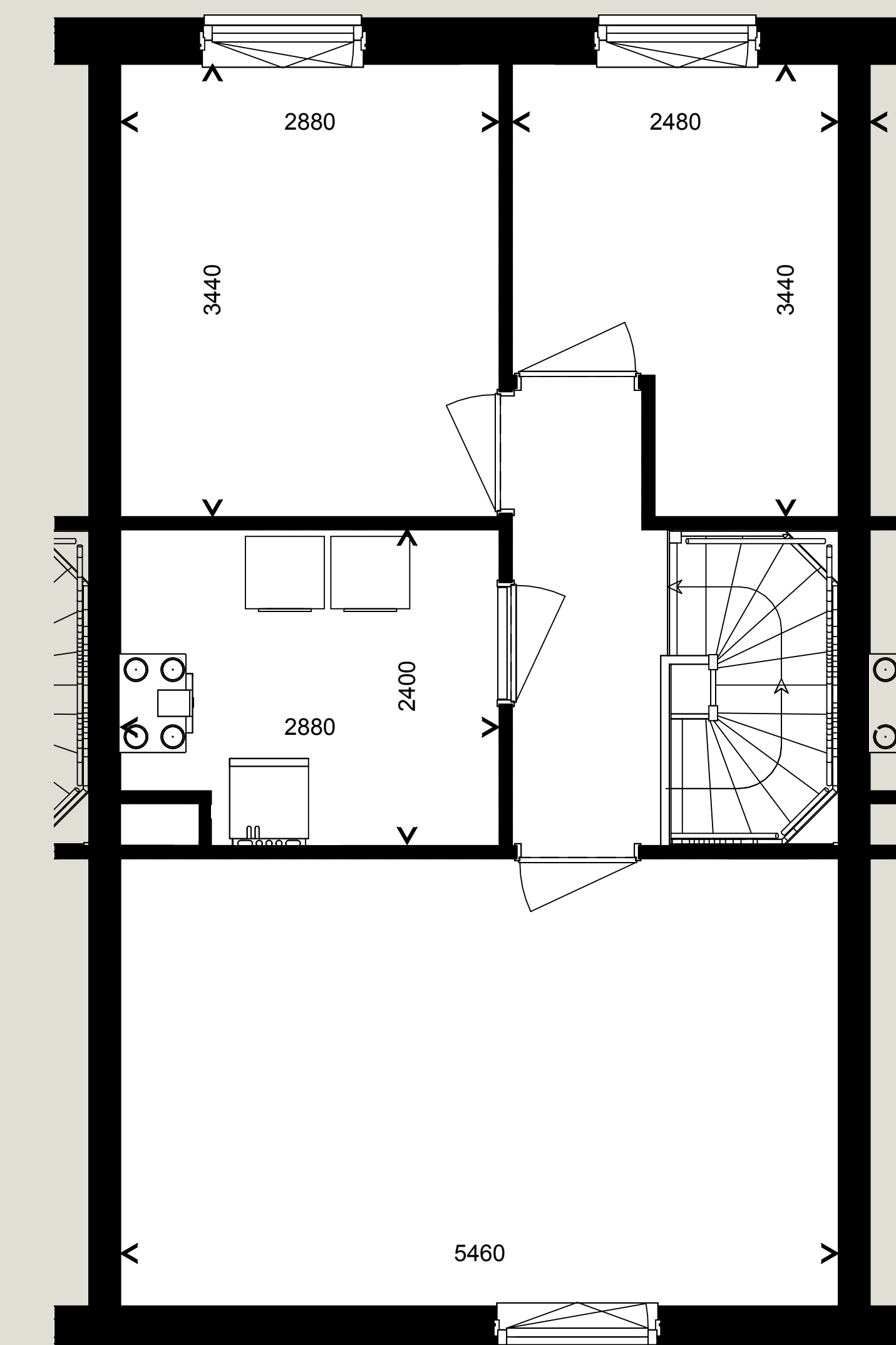
Derde verdieping
