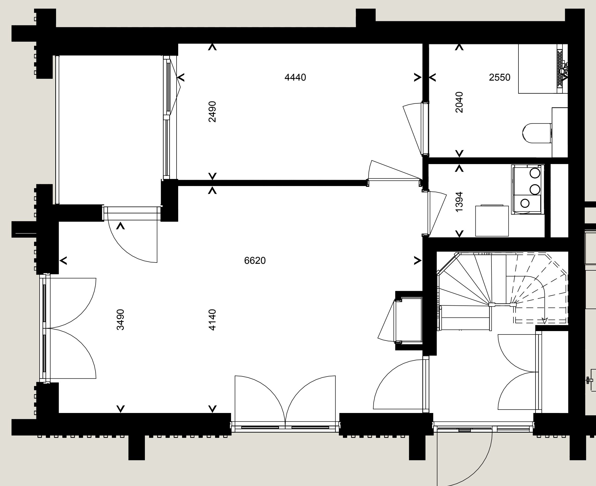
Begane grond
