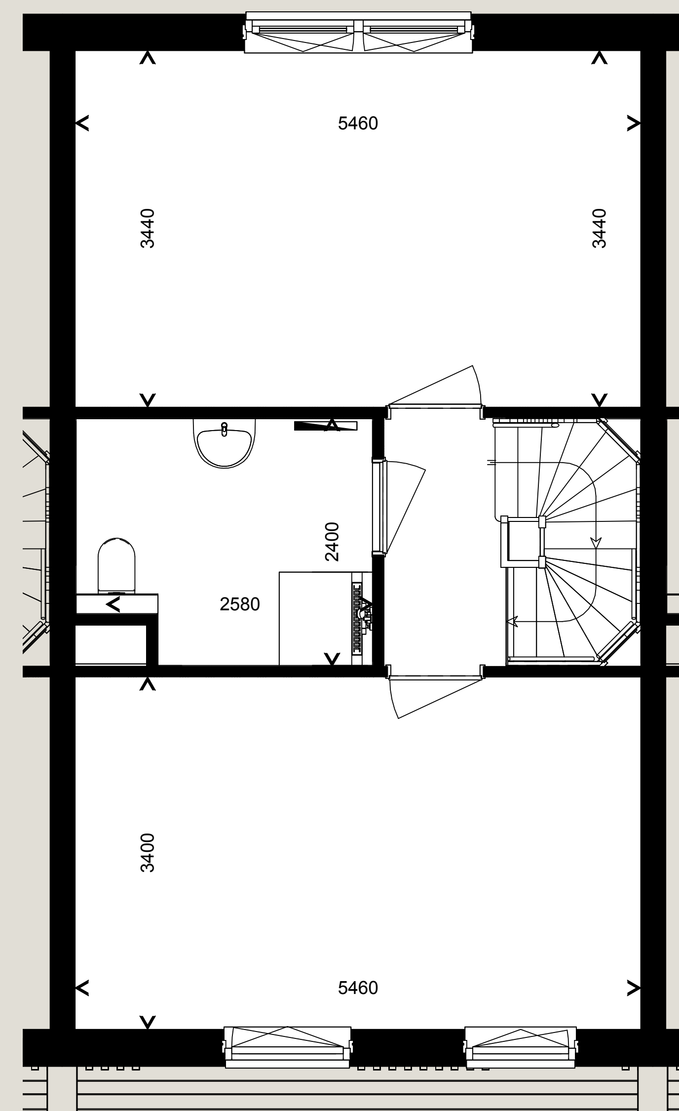
Eerste verdieping
