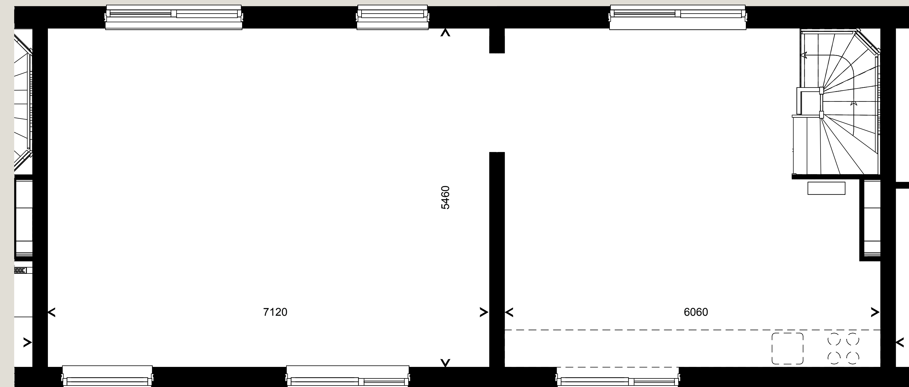
Tweede verdieping
