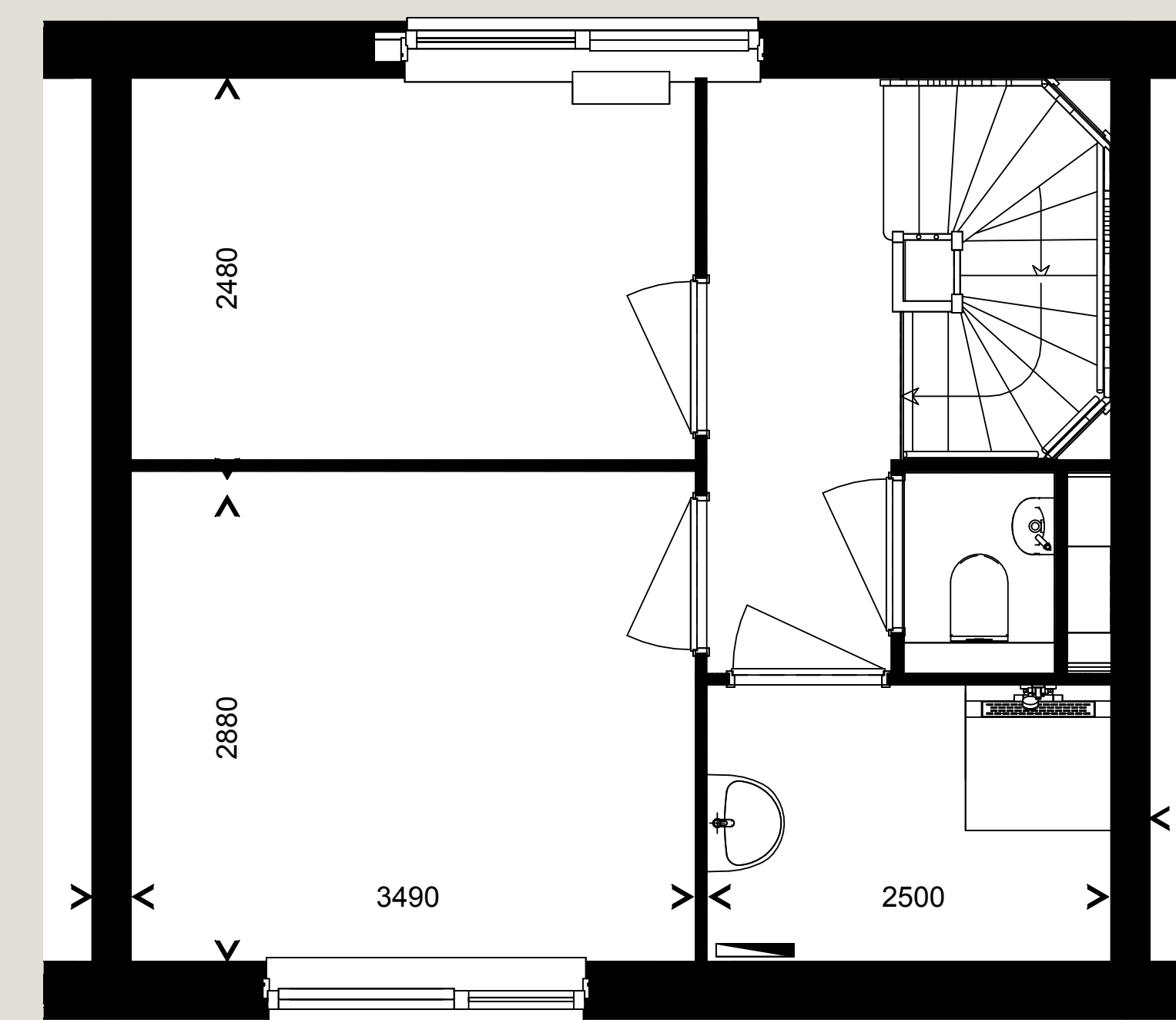
Tweede verdieping
