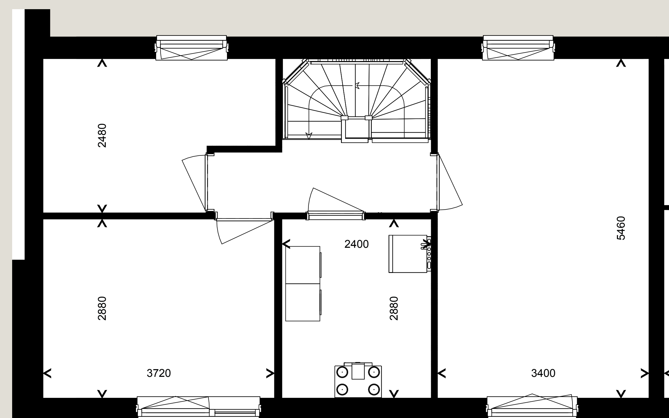
Derde verdieping
