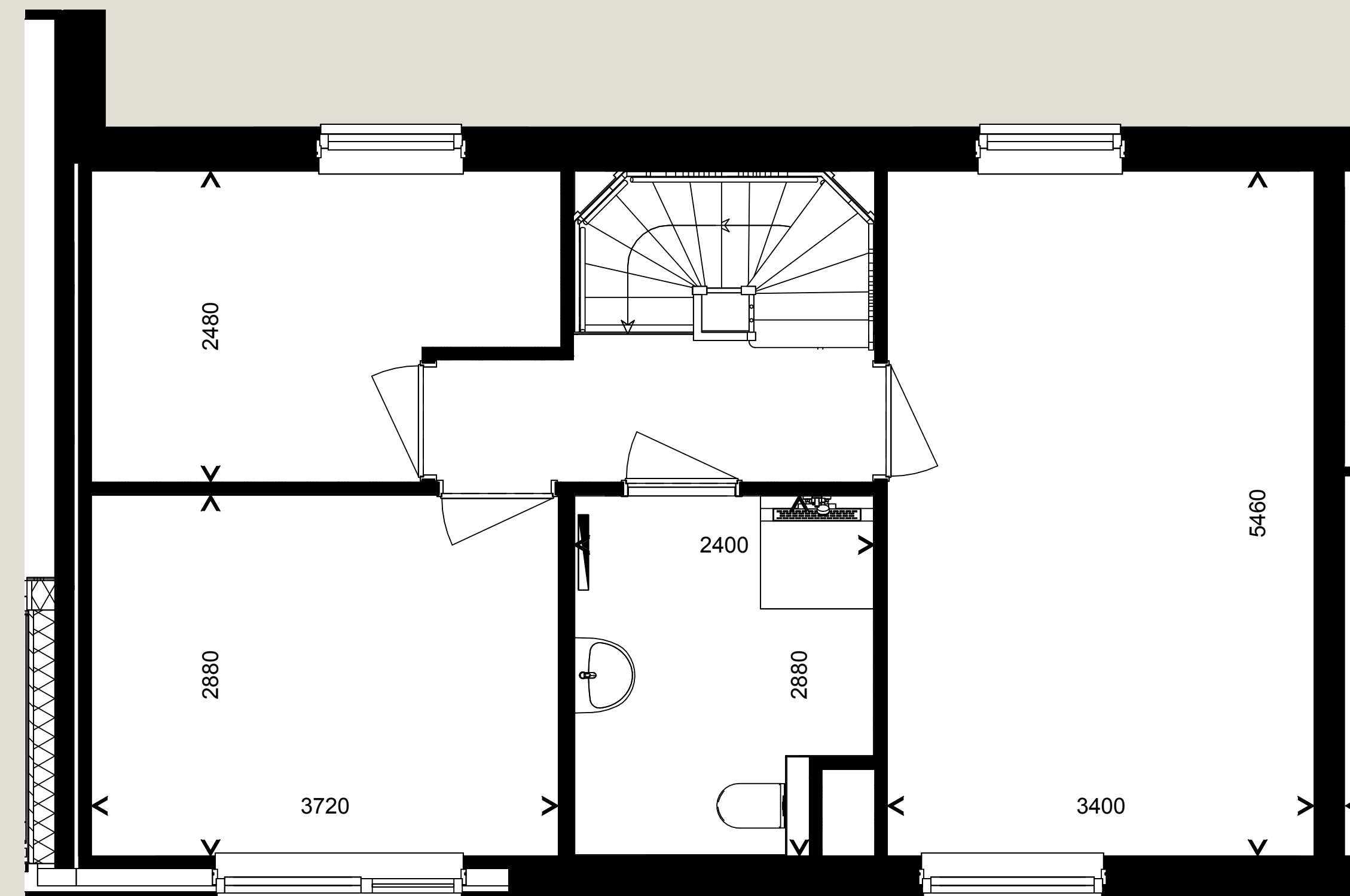
Tweede verdieping
