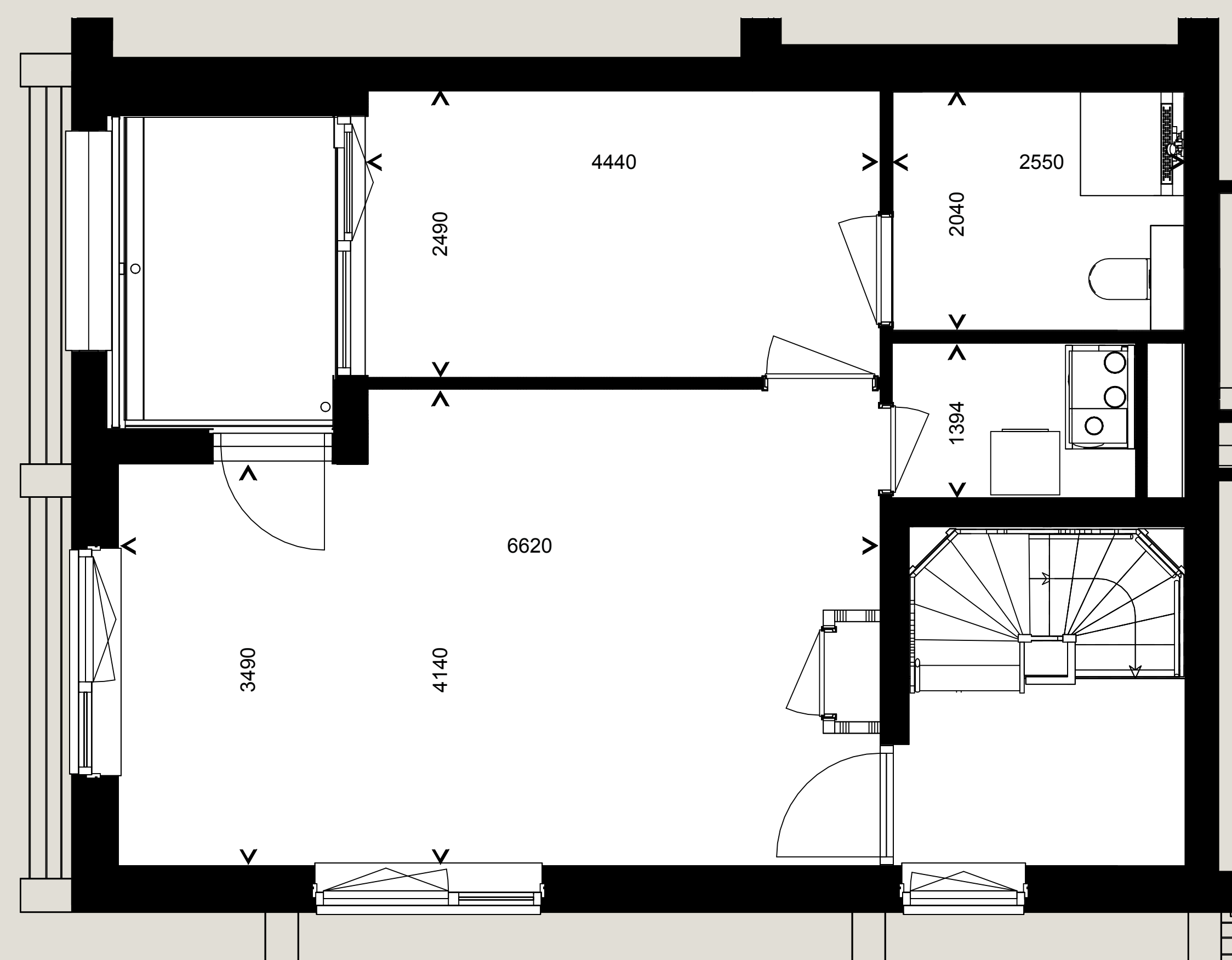
Eerste verdieping
