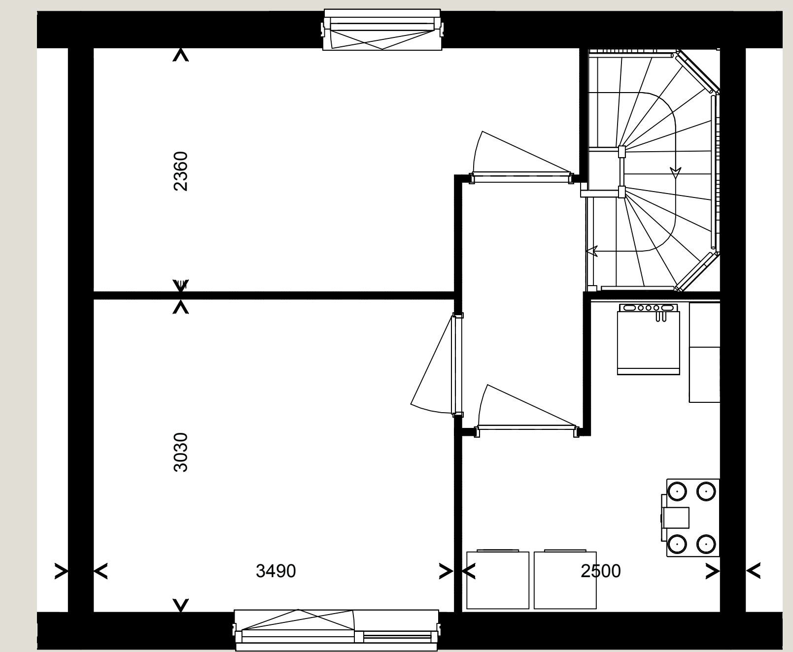
Derde verdieping
