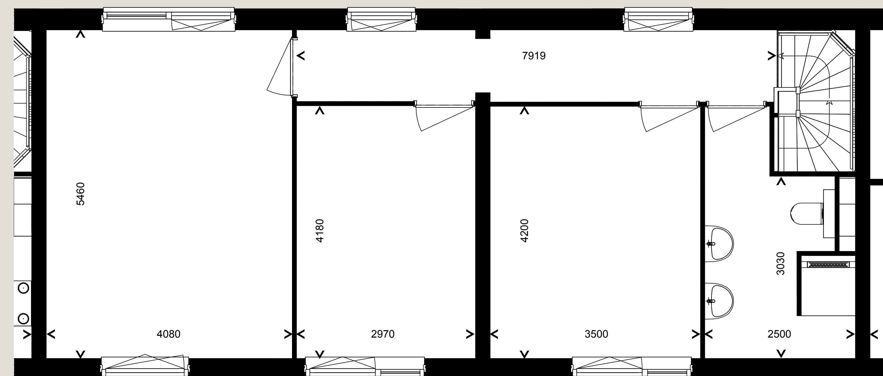
Derde verdieping
