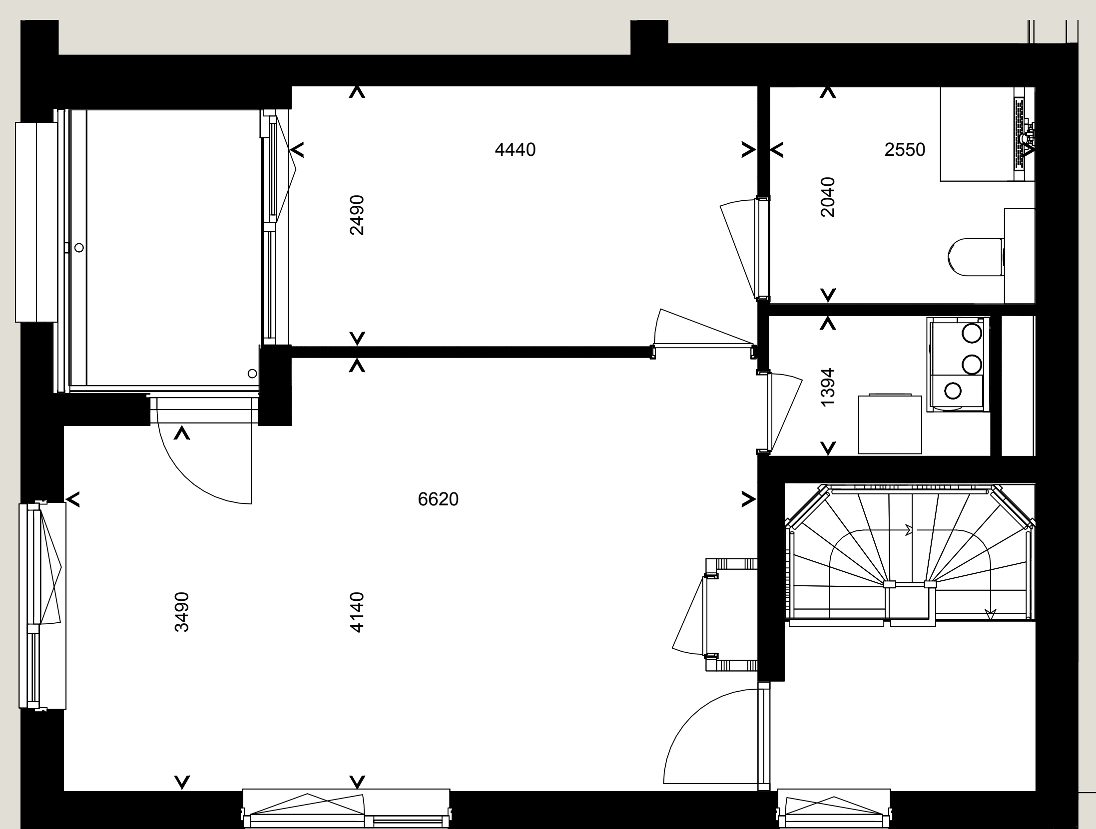
Derde verdieping Geldt alleen voor de bouwnummers 56 en 67 en 88
