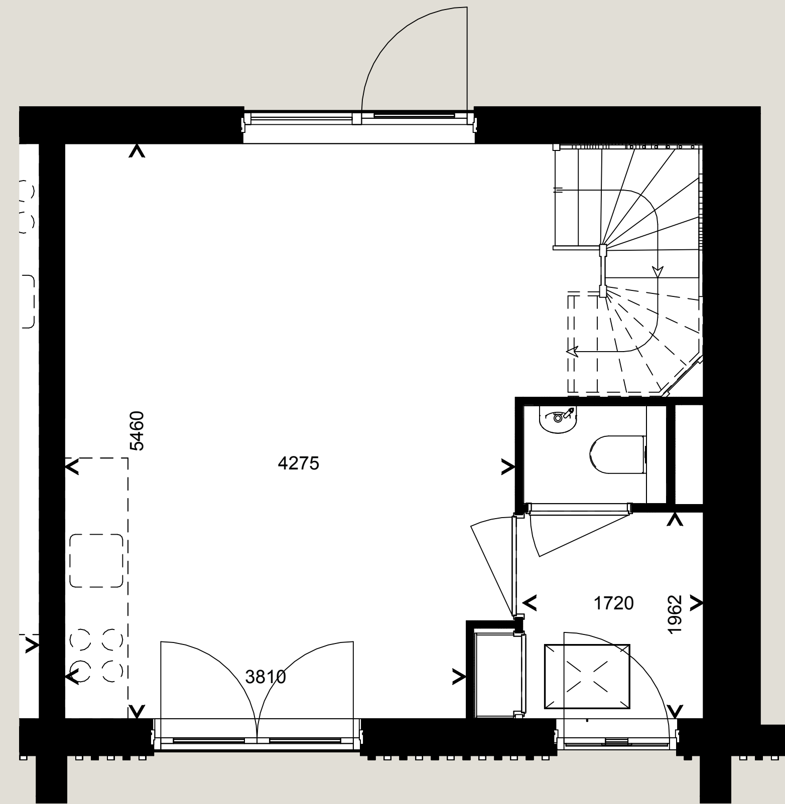
Begane grond
