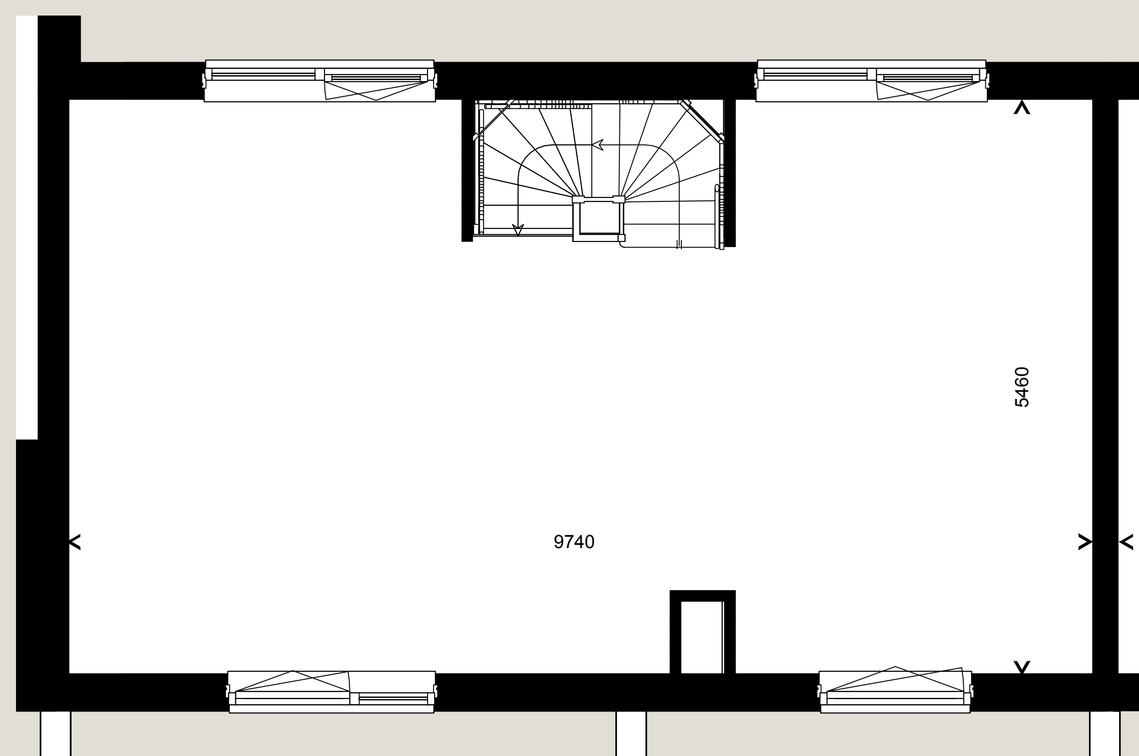
Eerste verdieping
