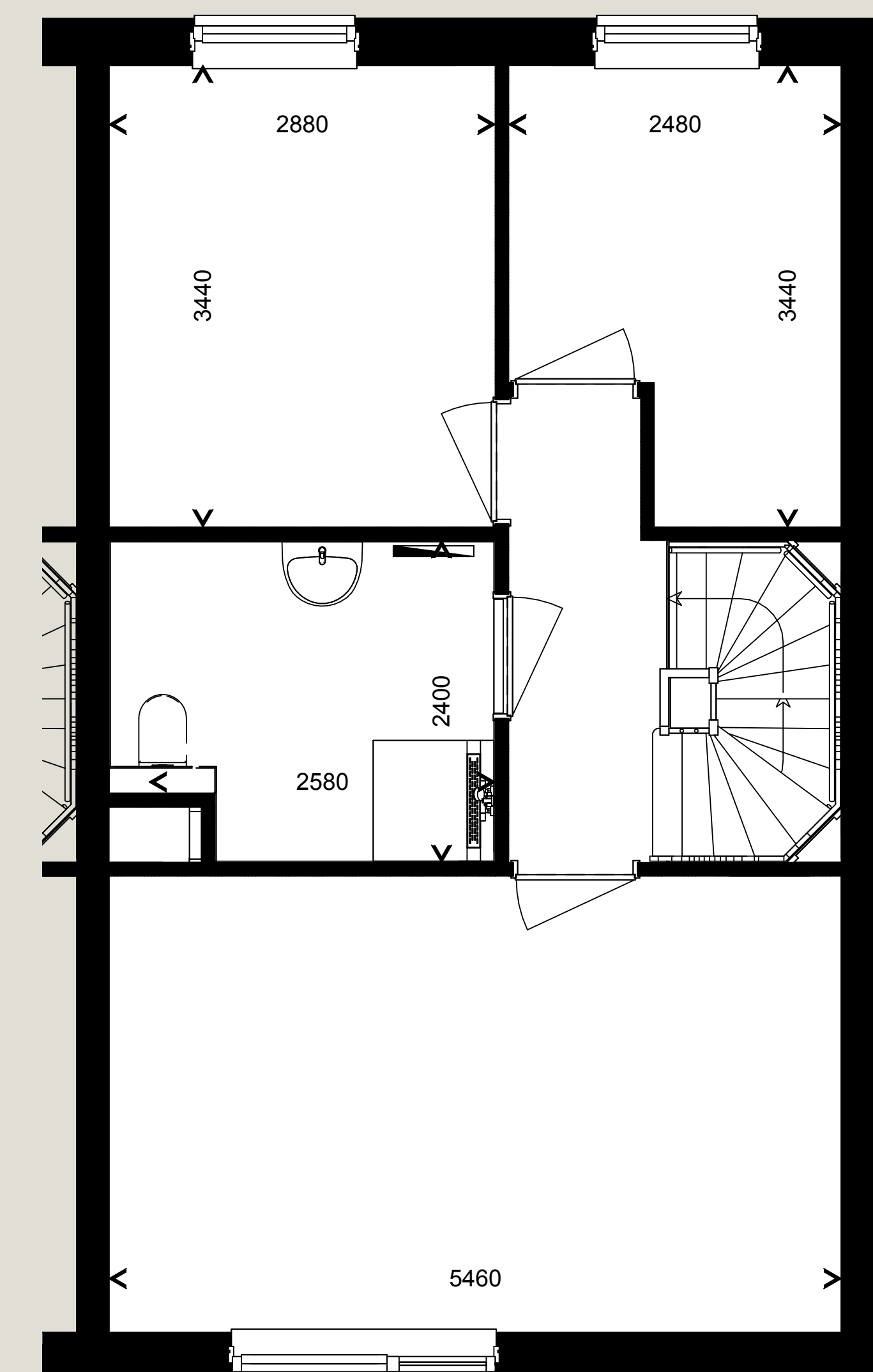
Tweede verdieping
