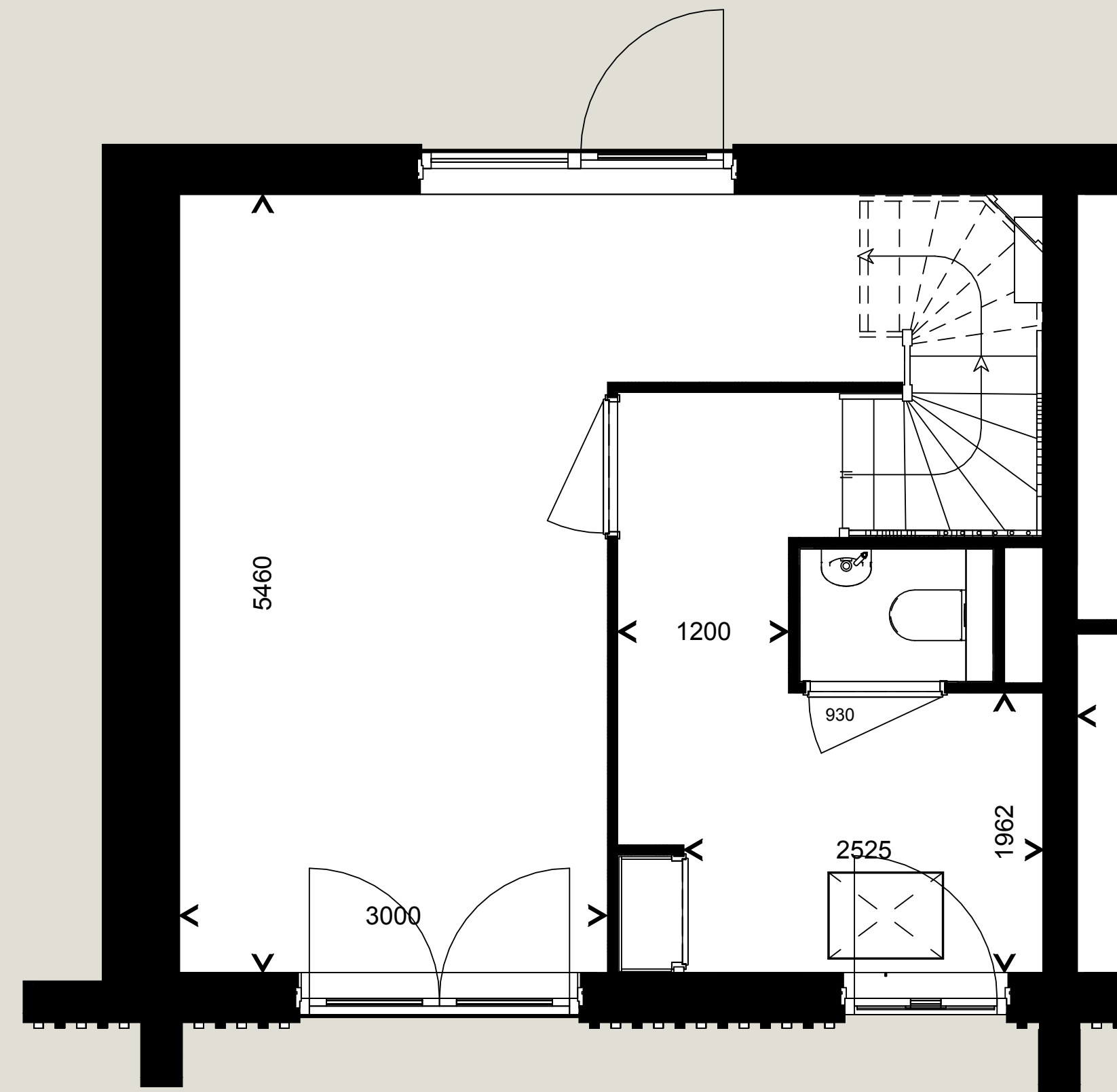
Begane grond
