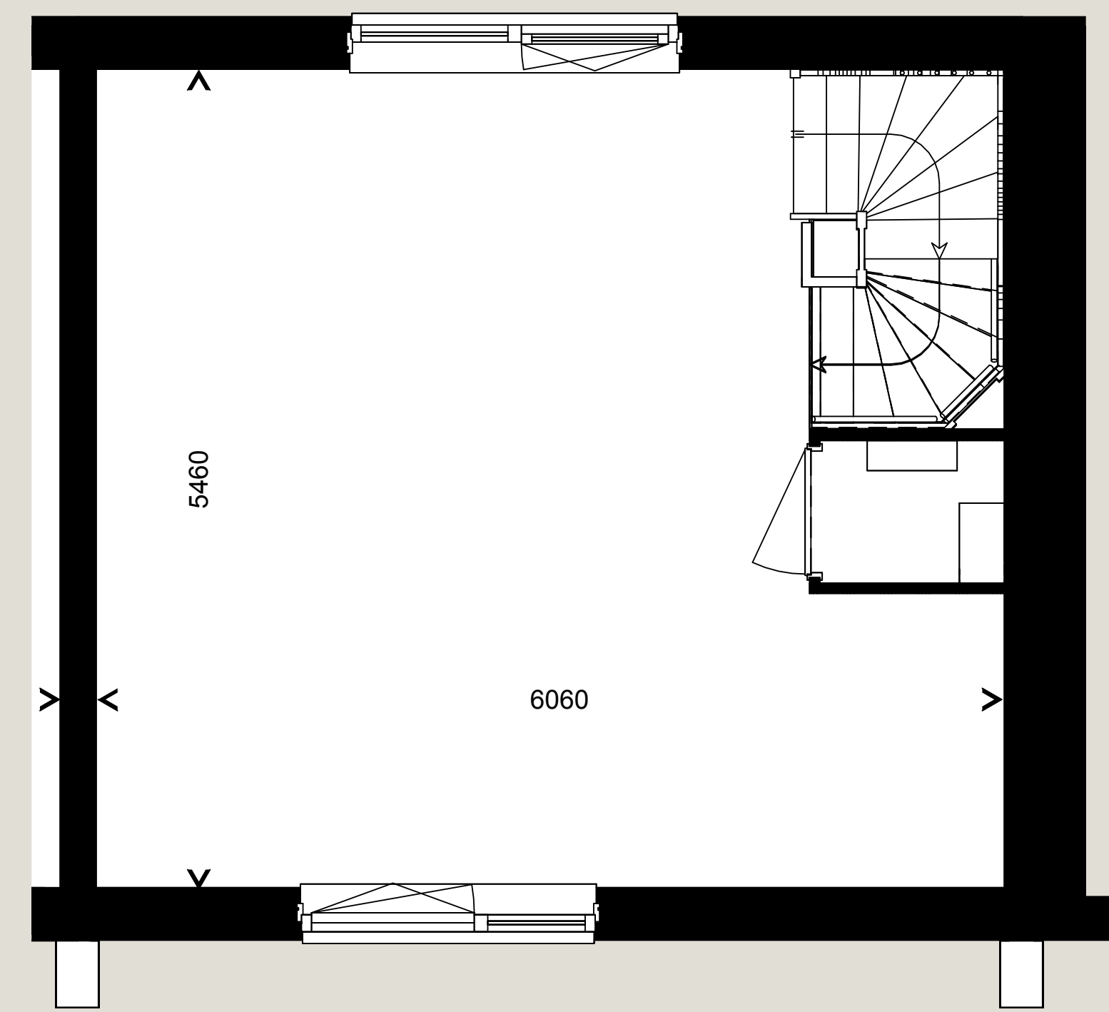
Eerste verdieping
