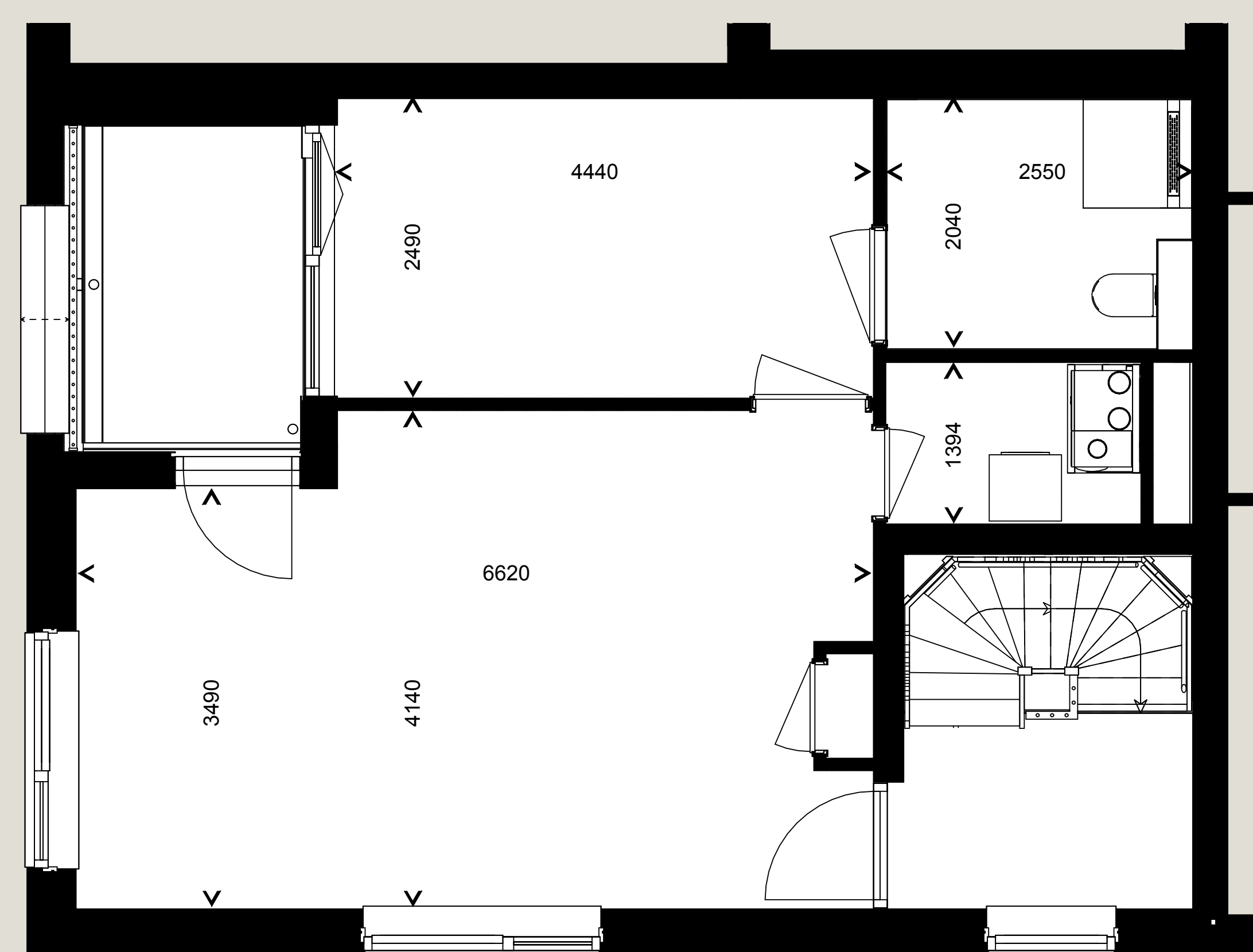
Tweede verdieping
