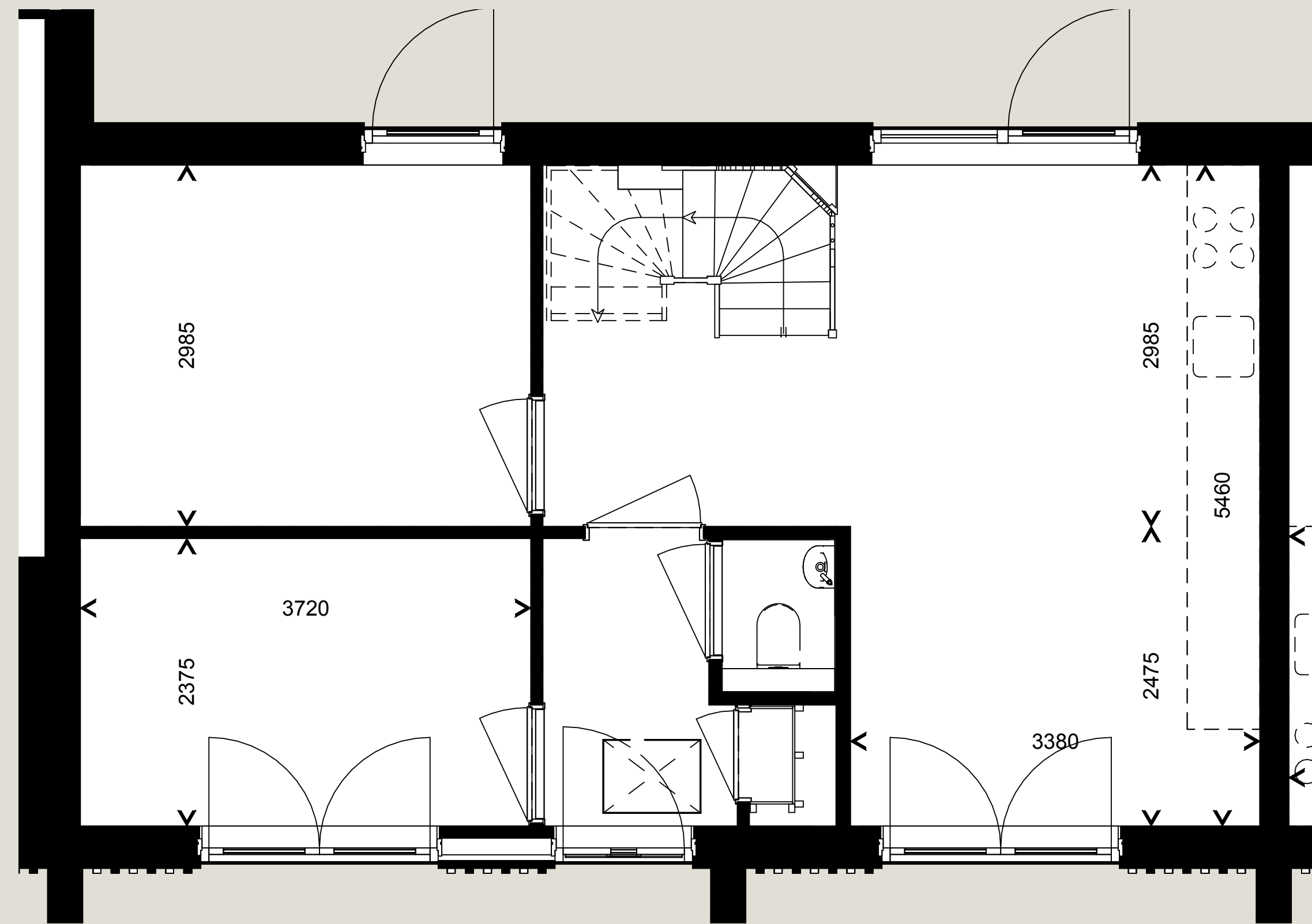
Begane grond
