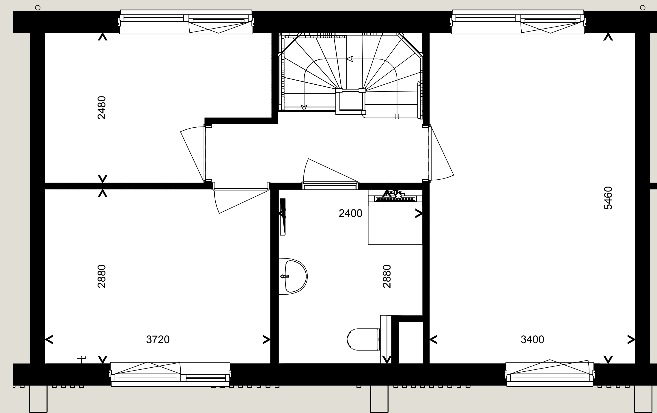
Eerste verdieping
