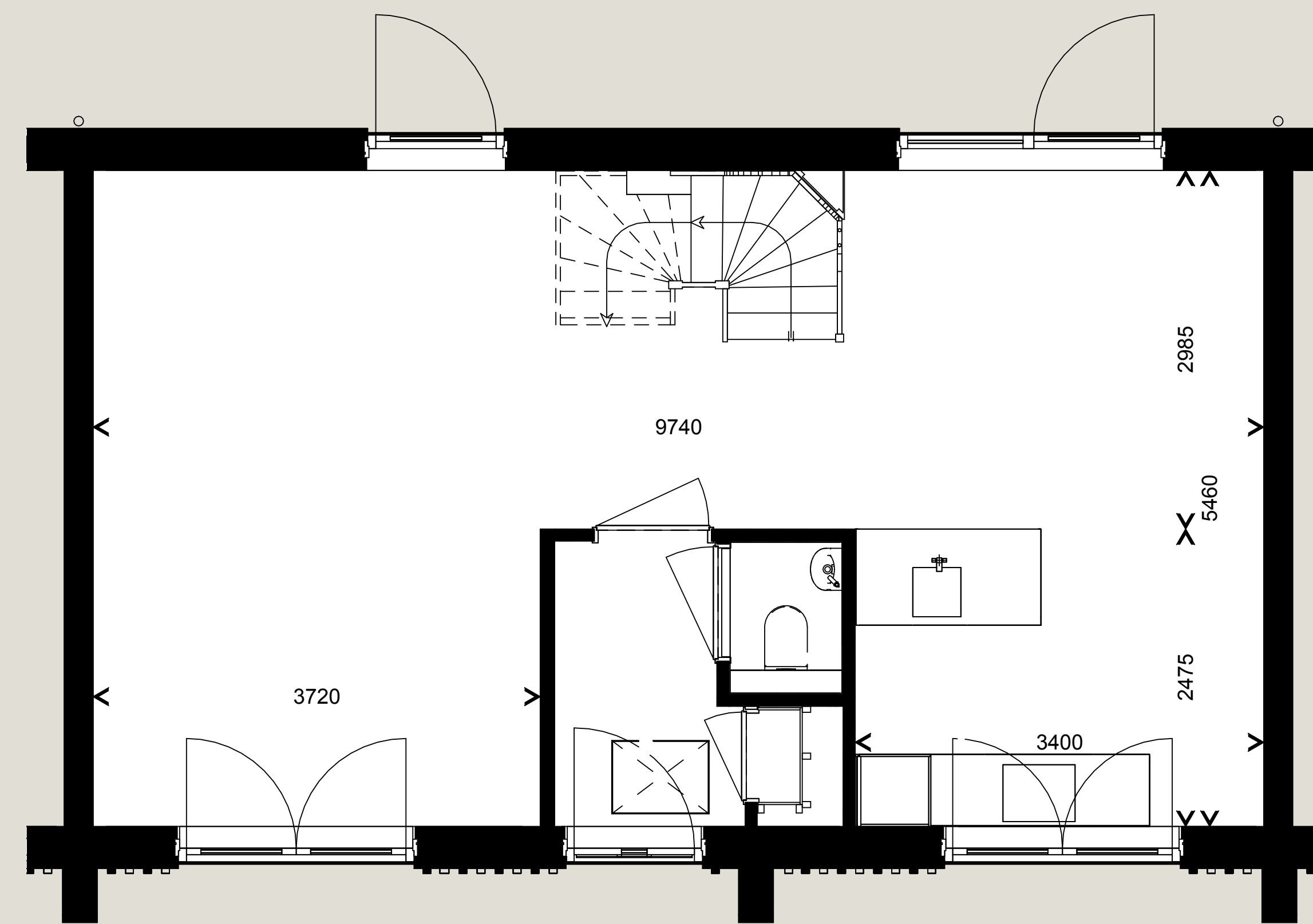
Begane grond
