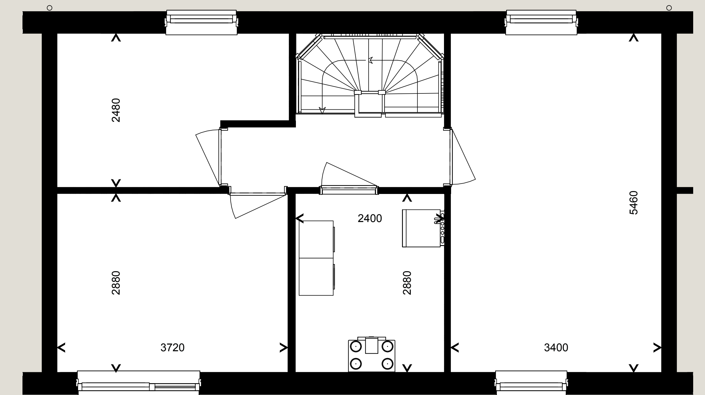
Tweede verdieping
