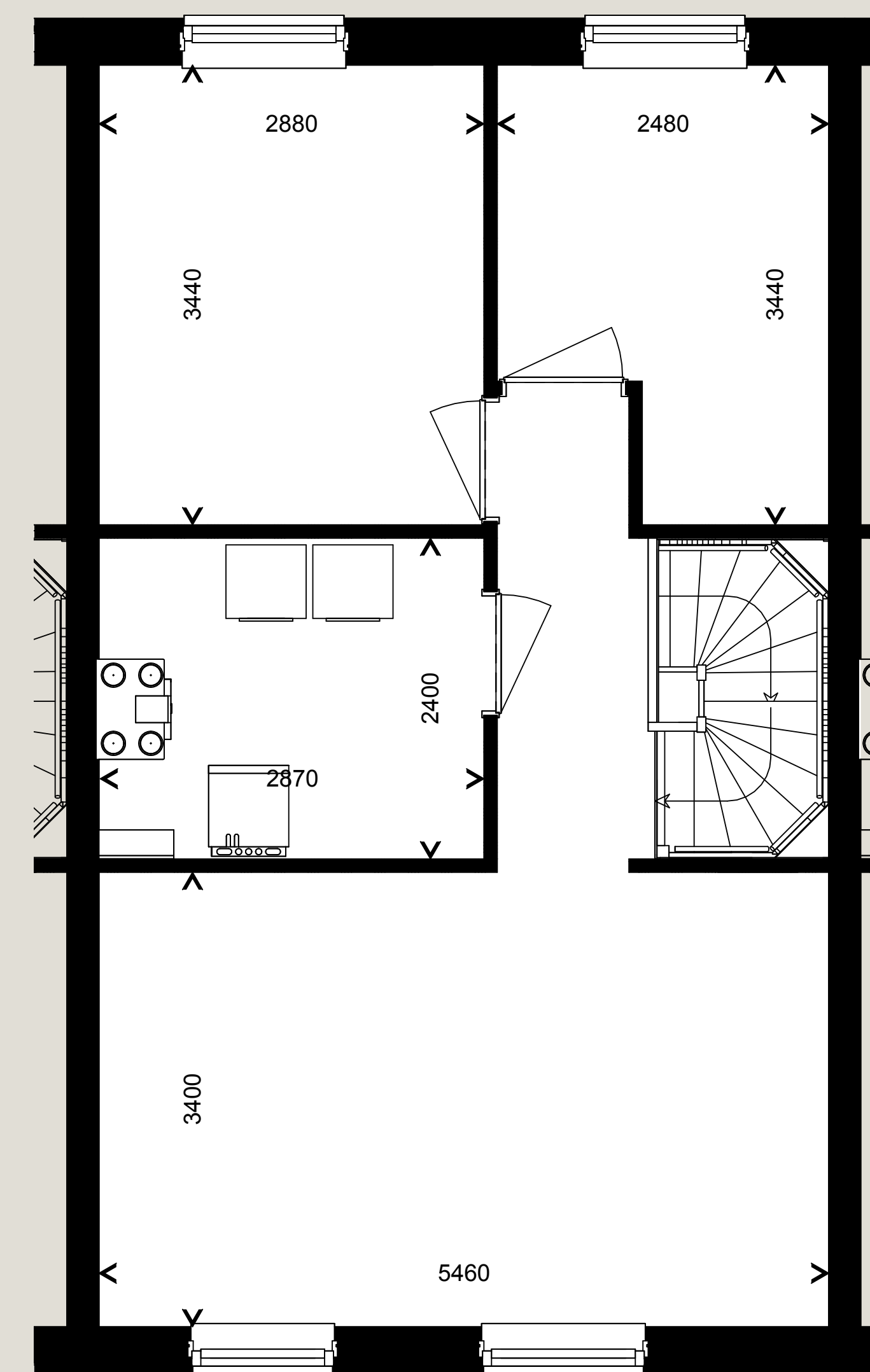
Tweede verdieping
